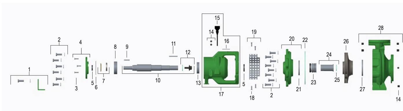
Figura 16 - Componentes da bomba
