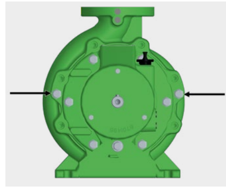
Figura 19 - Vista da tampa de pressão ilustrando parafusos
