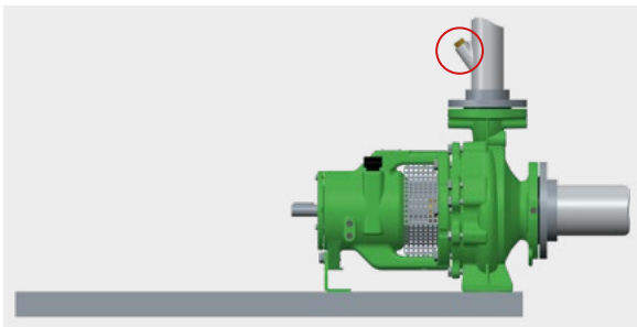
Figura 14 - Instalação bujão de escorva
