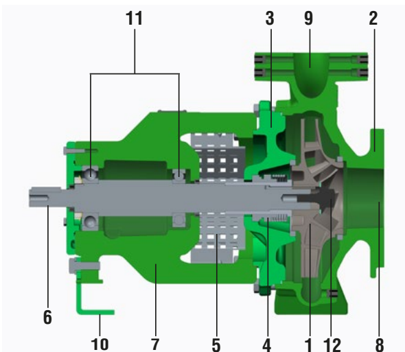
Figura 3 - Componentes
