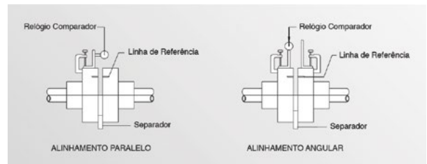
Figura 9 - Alinhamento do acoplamento usando relógio comparador.
