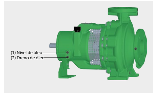
Figura 15 - Lubrificação
